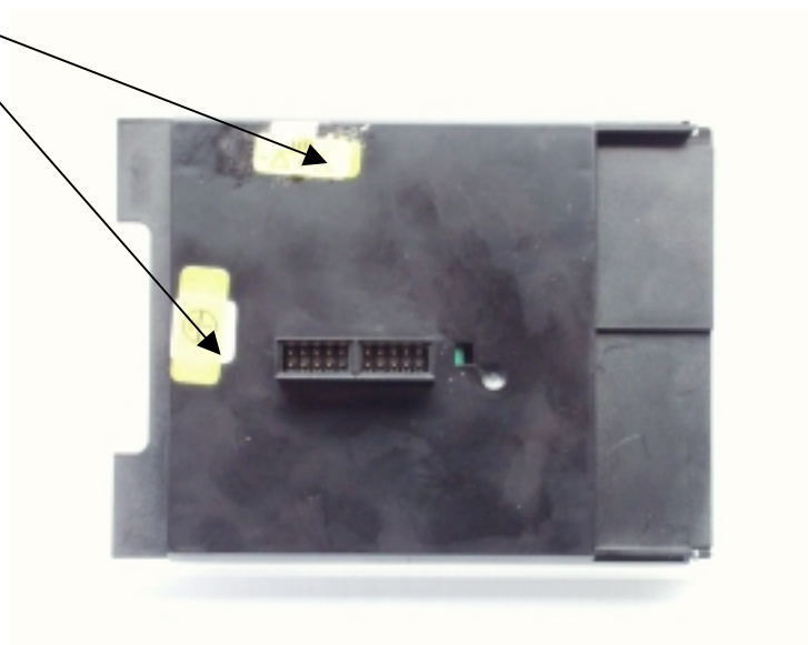
Slika 1: Zaštita od neovlaštena pristupa mjeriteljskim parametrima računске jedinice INFOCAL 5 nakon ovjeravanja
